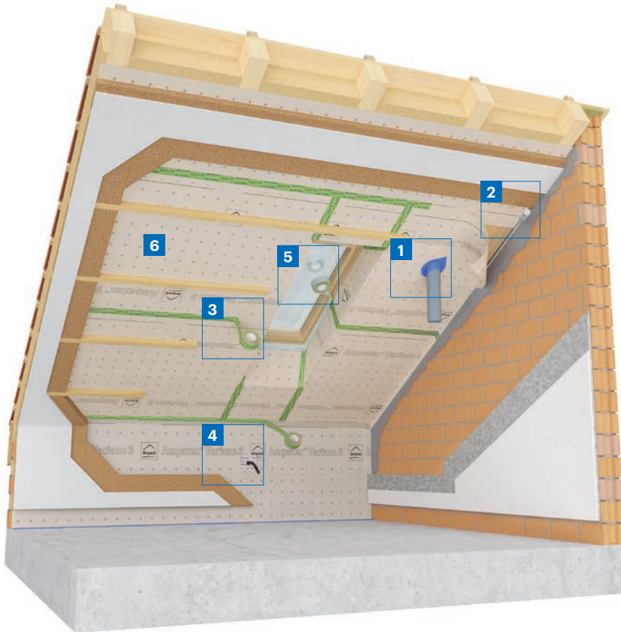
6 Ampatex® Variano 3 Moisture-variable vapour check and airtight layer
