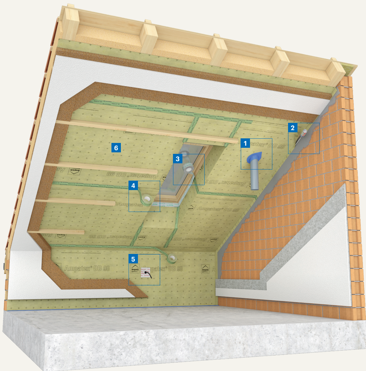
6 Freni vapore
