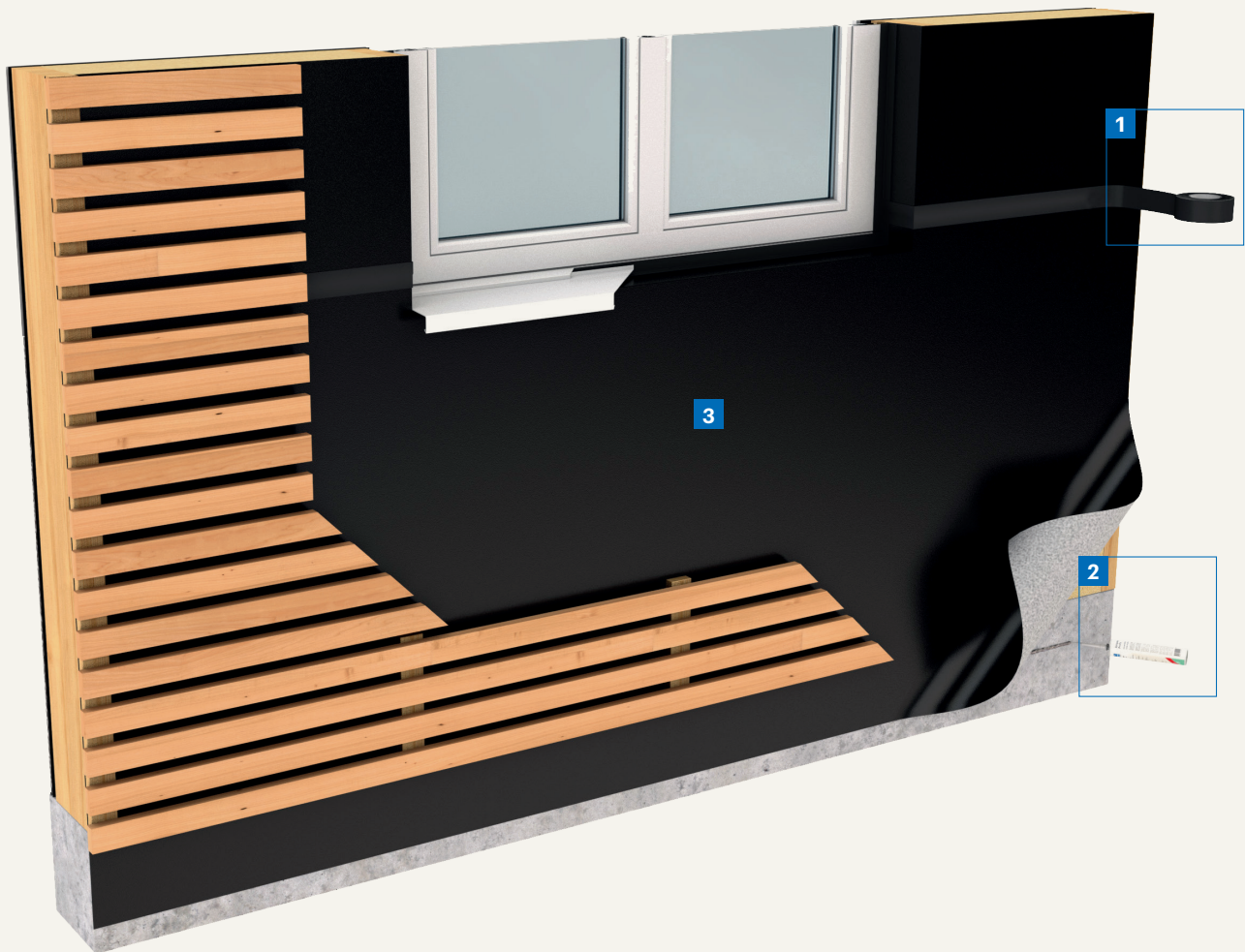
3 Wall membrane
