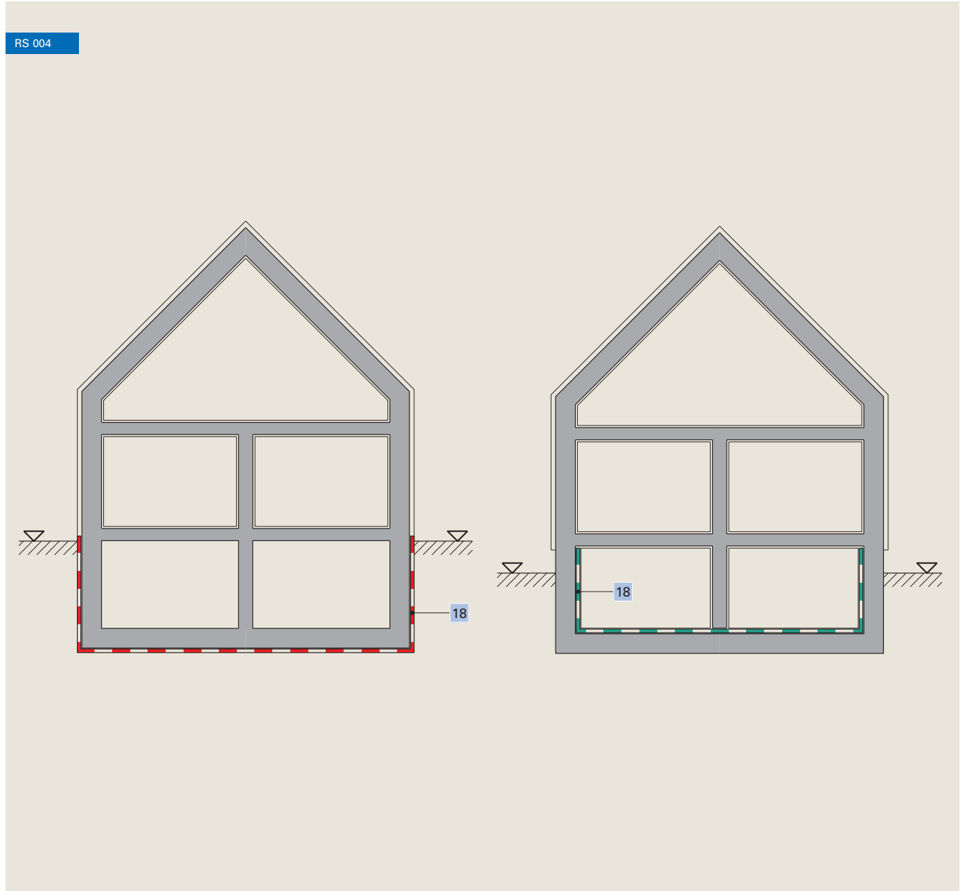
18 Radonsperre Sisalex® 871
